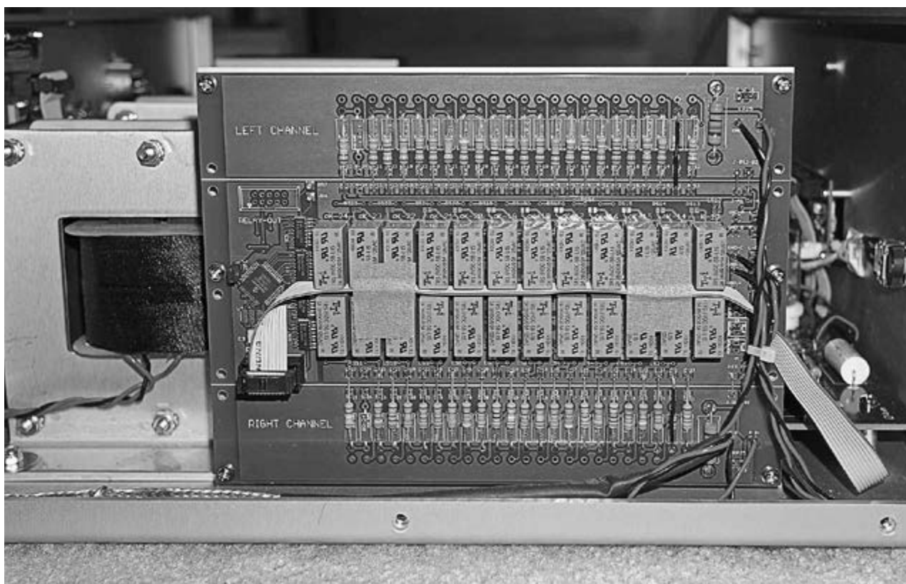
這是二十三級遙控音量掣 (Volume)，每聲道的音頻只經一粒 AUDIO NOTE 用開過的 Tantalum 電阻。
